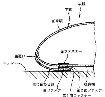
図4 面ファスナーの契合状態断面図
