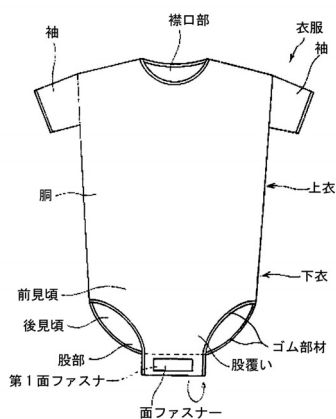
図1 衣服の下衣部の股部を開放状態の正面図
