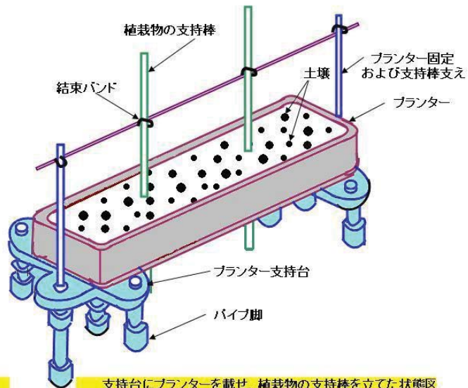
支持台にプランターを載せ、植栽物の支持棒を立てた状態図
