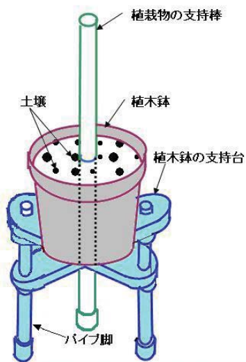
支持台に鉢を載せ、植栽物の支持棒を立てた状態図
